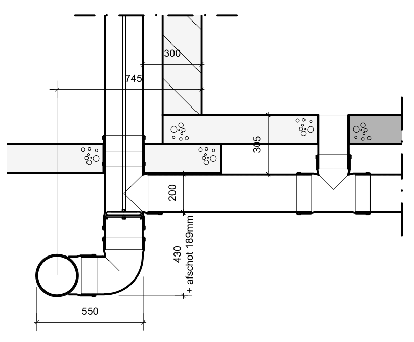
aftapbuis met mestkanaal
