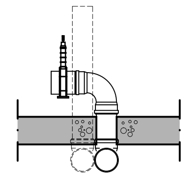
afsluiter waterkanaal spoelleiding
