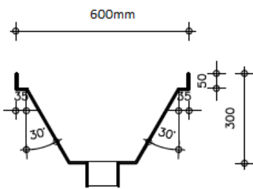
doorsnede A-A
